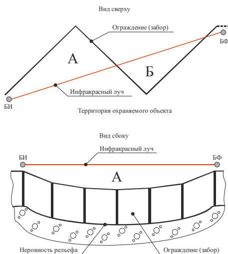
Рисунок 65 – Пример неправильного размещения ИК извещателя
