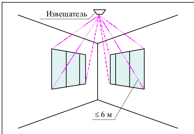
Рисунок 19 – На потолке (вариант 2)
