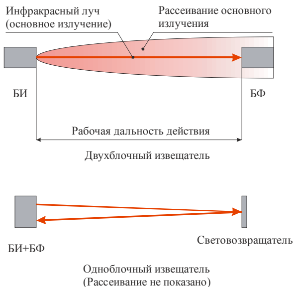
Рисунок 64 – Пример активного ИК извещателя
