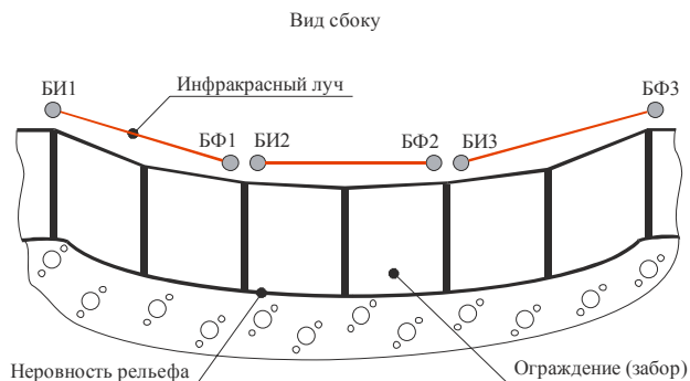
Рисунок 66 – Пример охраны объекта криволинейной формы
