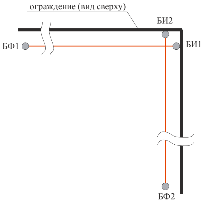
Рисунок 77 – Пример блокировки ограждения, имеющего излом
