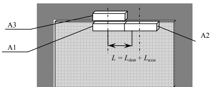
Рисунок 11 – Схема размещения мест монтажа извещателя и ДВМП
