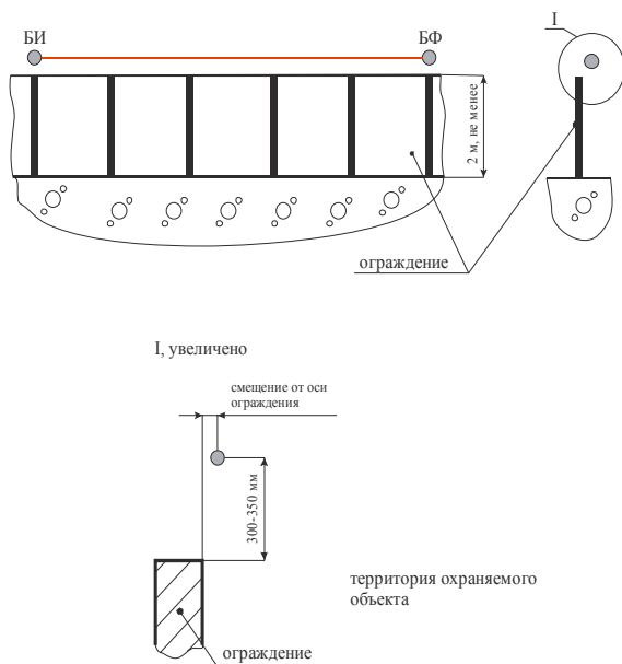
Рисунок 76 – Пример блокировки ограждения
