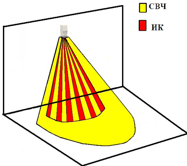
Рисунок 101 – Зона обнаружения извещателя «Сокол-2»
