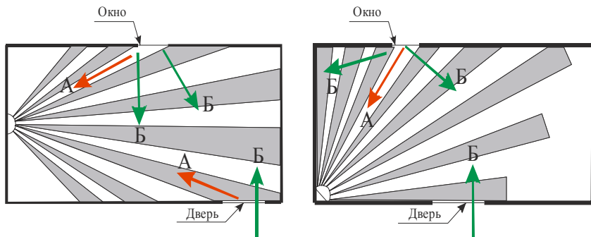
Рисунок 41 – Возможные траектории перемещения нарушителя в зоне обнаружения ИК извещателя, устанавливаемого на стене
