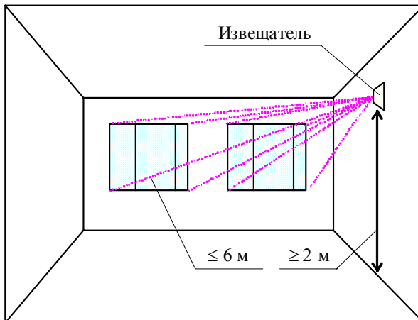
Рисунок 16 – На боковой стене
