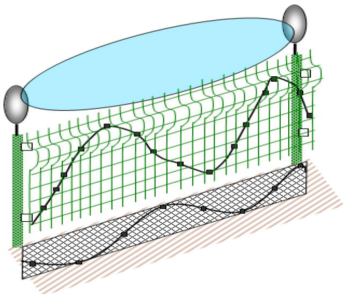
Рисунок 121 – Установка извещателя «Рубеж» на стальной сварной сетке
