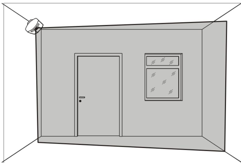
Рисунок 107 – Установка извещателя с поверхностной зоной обнаружения в угол общего проема
