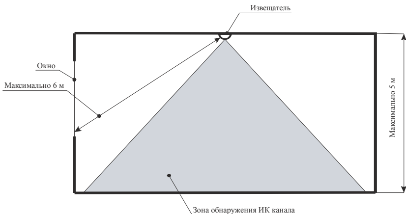
Рисунок 110 – Установка извещателя конусообразной ЗО на потолке охраняемого помещения (вид сбоку)
