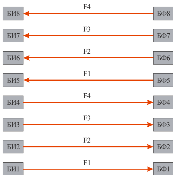
Рисунок 67 – Пример ИК барьера со встречно направленными лучами
