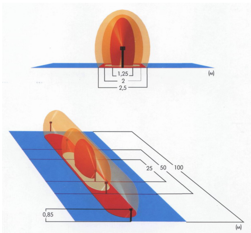
Рисунок 92 – Зоны обнаружения извещателя «Линар-200»
