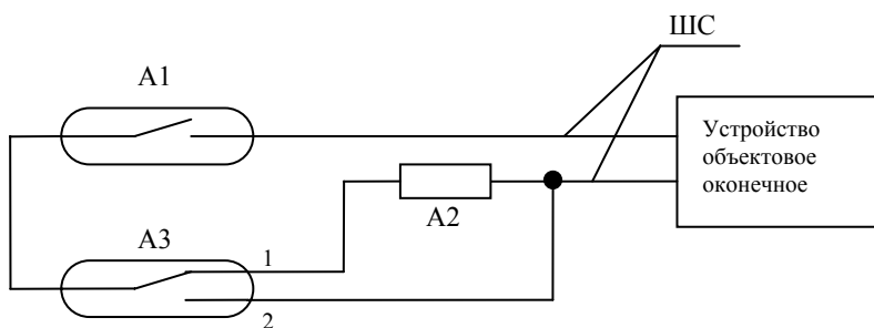
Рисунок 9 – Схема защиты магнитоcontactного извещателя от саботажа
