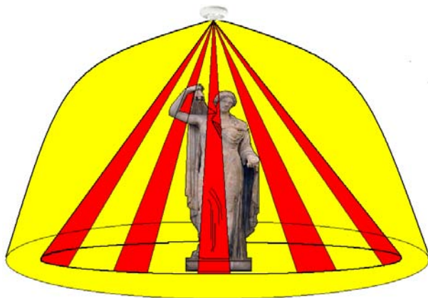
Рисунок 102 – Зона обнаружения извещателя «Сокол-3»
