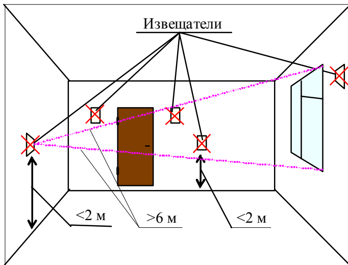
Рисунок 21 – Не рекомендуемые места установки извещателя
