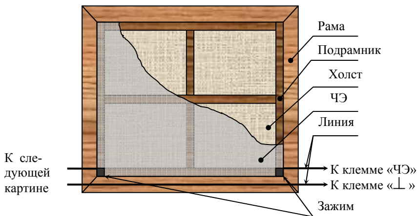
Рисунок 95 – Пример охраны картины емкостным извещателем
