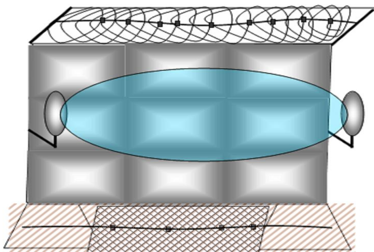
Рисунок 120 – Установка извещателя «Рубеж» на бетонном заграждении
