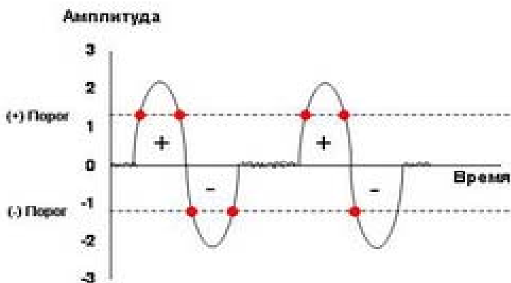
Рисунок 98 – Пример принципа работы ИК извещателя
