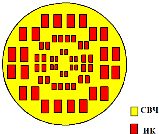
Рисунок 103 – Проекция трех зон обнаружения извещателя «Сокол-3»
