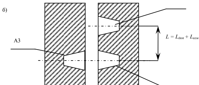
Рисунок 10 – Схема размещения мест монтажа извещателя и ДВМП
