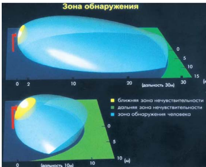
Рисунок 86 – Зоны обнаружения извещателя.
