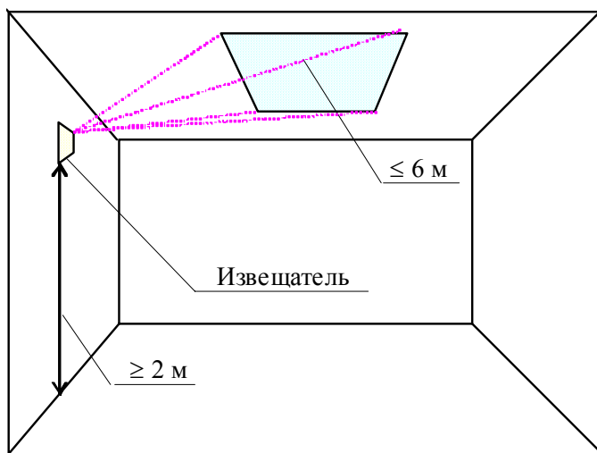
Рисунок 20 – На боковой стене (охрана остекленного перекрытия)
