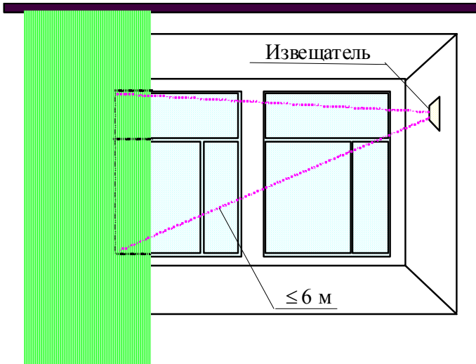
Рисунок 15 – Между стеклом и жалюзи
