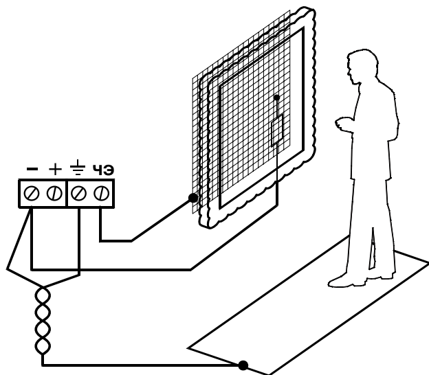
Рисунок 97 – Пример охраны картины при отсутствии на объекте шины заземления
