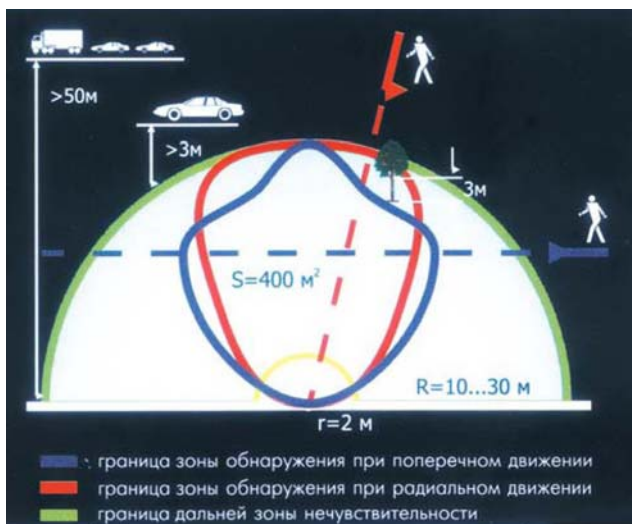
Рисунок 87 – Обнаружение при перемещениях по любым траекториям
