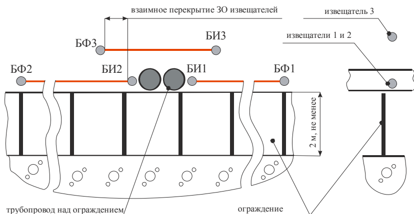
Рисунок 78 – Пример блокировки ограждения с конструкциями над ним
