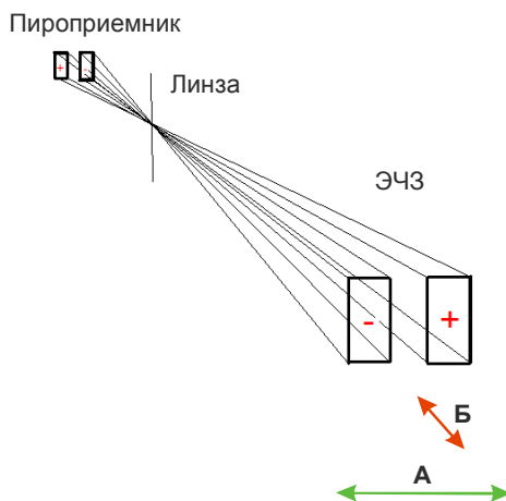
Рисунок 40 – Оптическая система ИК извещателя
