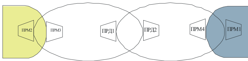
Рисунок 94 – Пример правильной последовательности включения линейных извещателей
